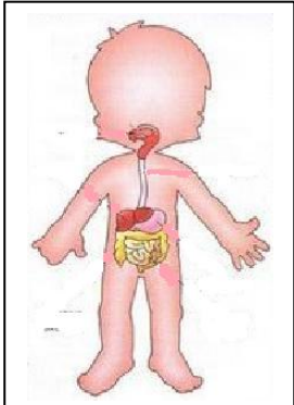
Aparell digestiu
