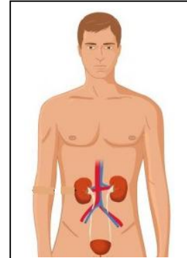
Aparell excretor
